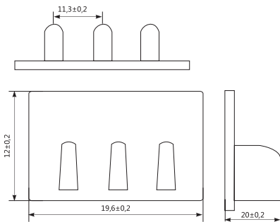
Заглушка на 4-полюсную шину
